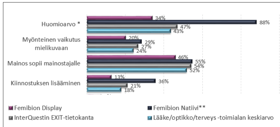
Kampanjatulostaulukko (Interquest)
